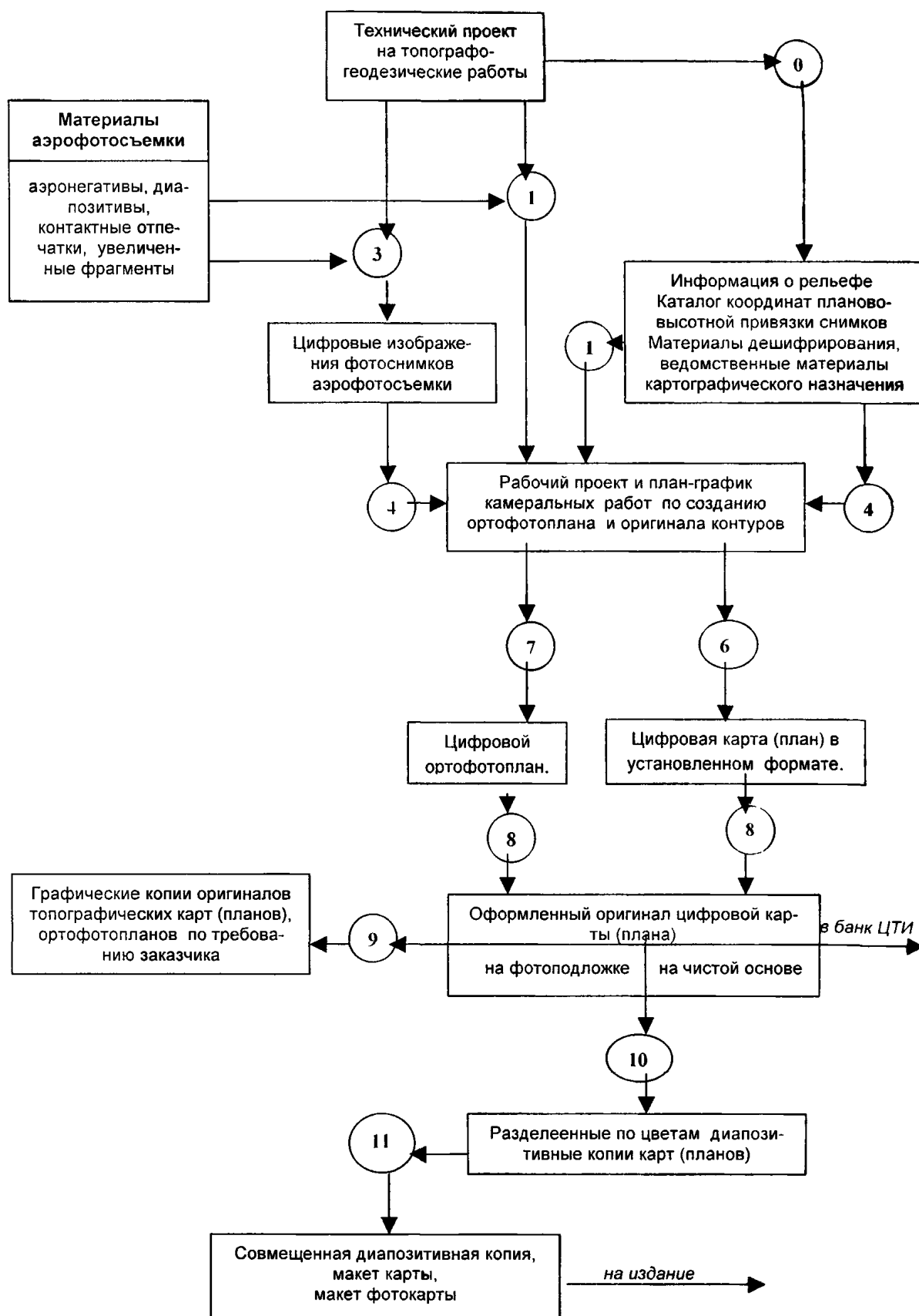
Рис. 4. Технологическая схема камеральных работ при комбинированной топографической съемке в масштабах 1:500 - 1:25 000 с использованием цифровых фотограмметрических приборов
