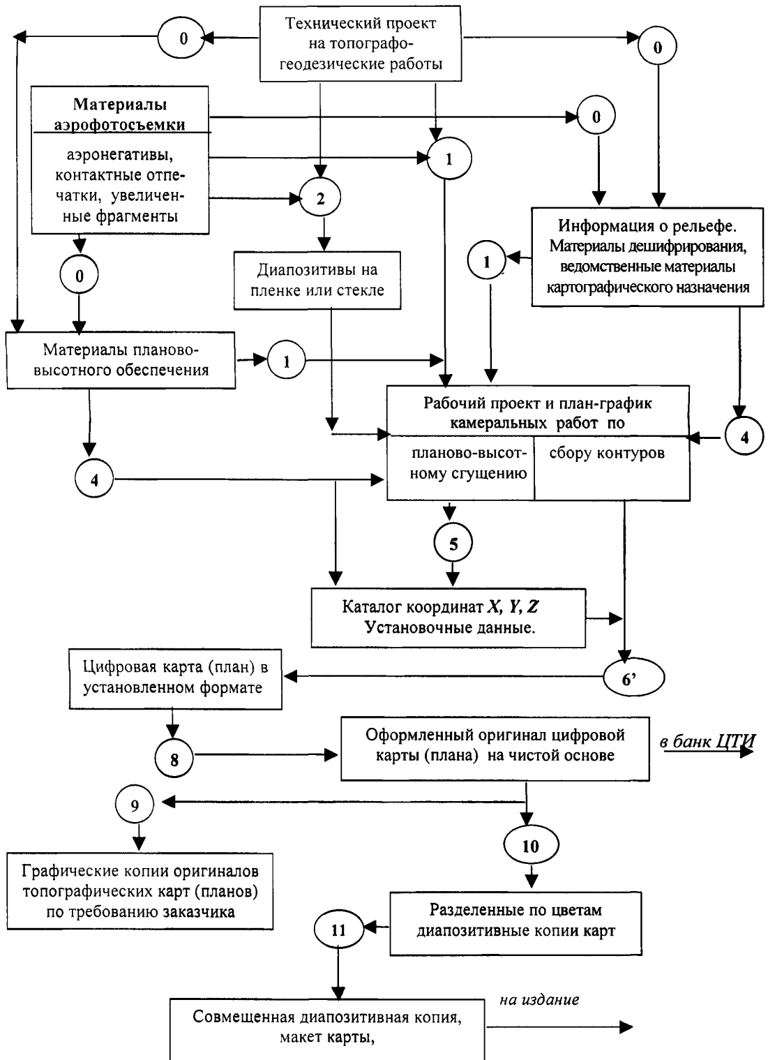
Рис. 5. Технологическая схема камеральных работ при комбинированной топографической съемке в масштабах 1:500 - 1:25000 с использованием аналитических фотограмметрических приборов
