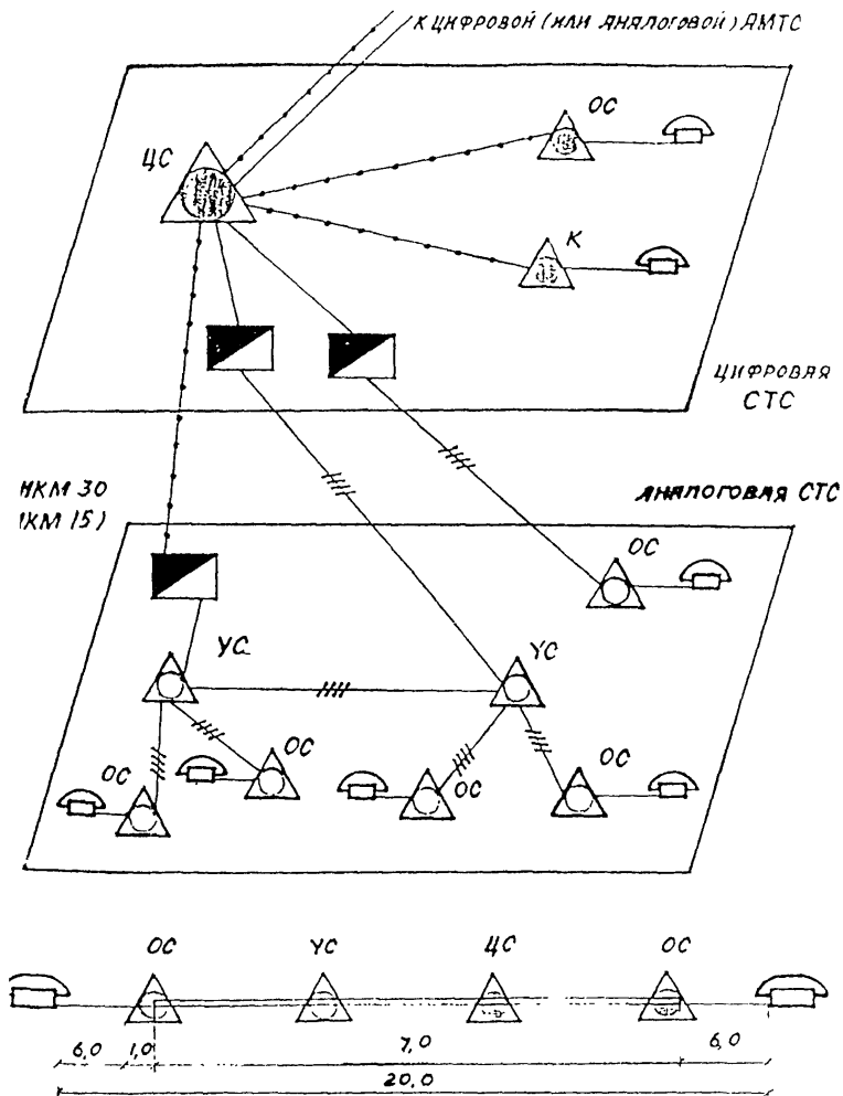
Рис. 2. Внедрение цифровых АТС на сельских телефонных сетях при демонтаже бывшей ЦС
