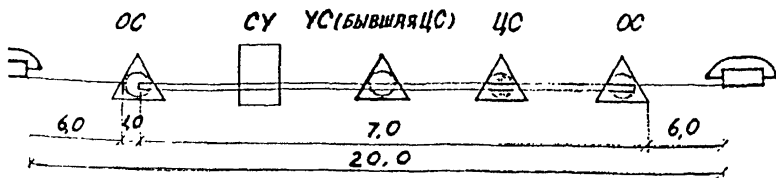
Рис. 1. Включение цифровых АТС на сельских телефонных сетях при переводе бывшей ЦС в ранг УС
