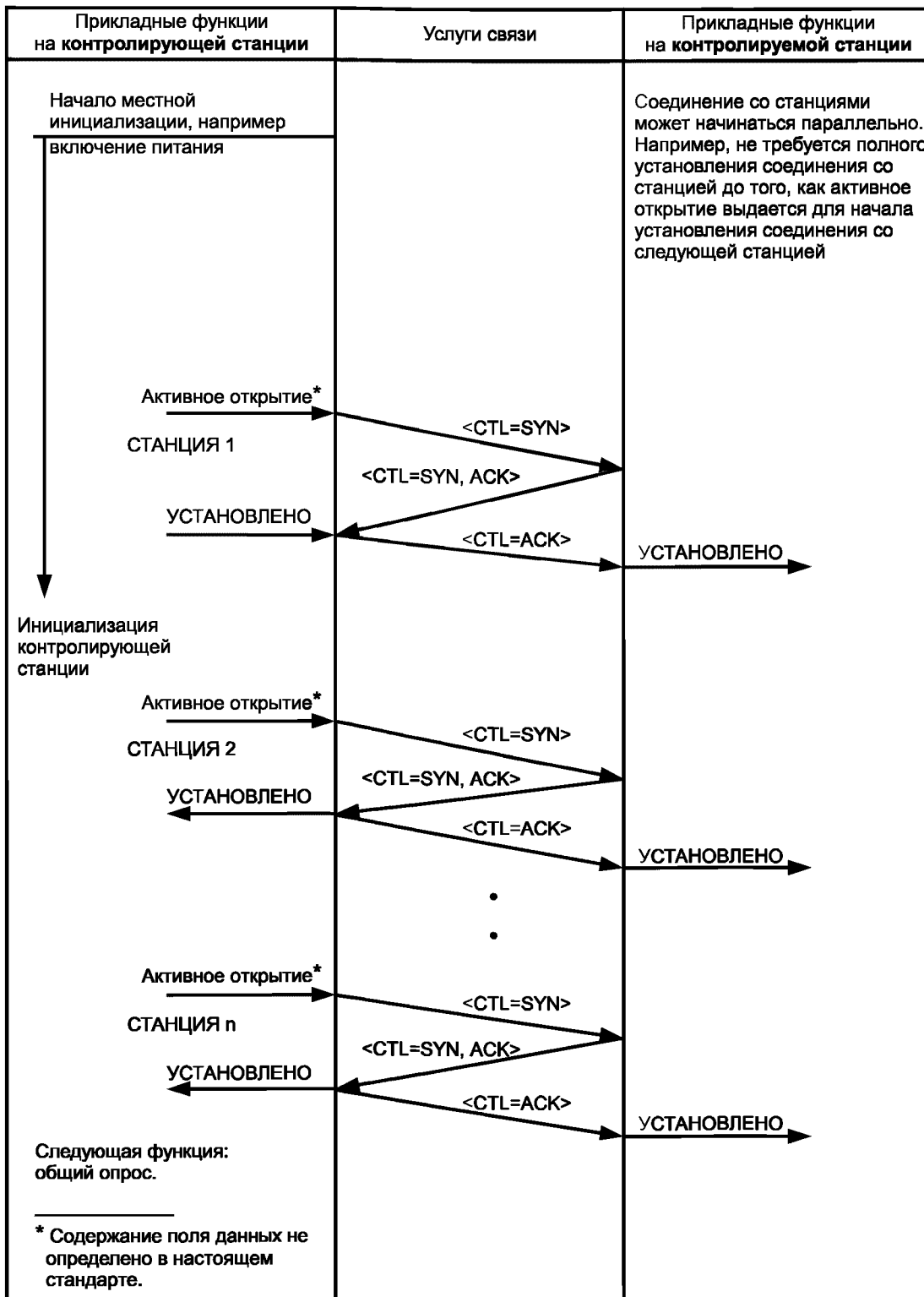
Рисунок 18 — Инициализация контролирующей станции
