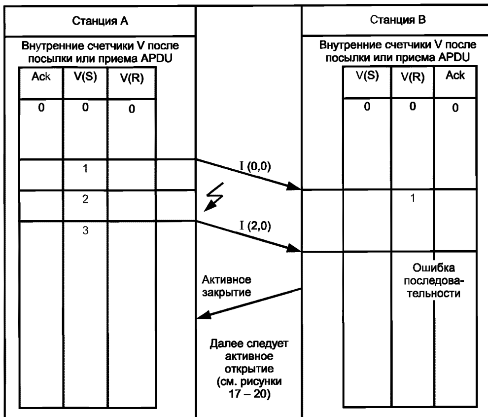
Рисунок 11 — Ненарушенная последовательность нумерованных APDU формата I
