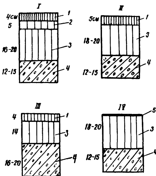
Рис.1. Типы конструкций дорожных одежд с основаниями из битумоминеральных смесей для дорог 1-IV категории:
