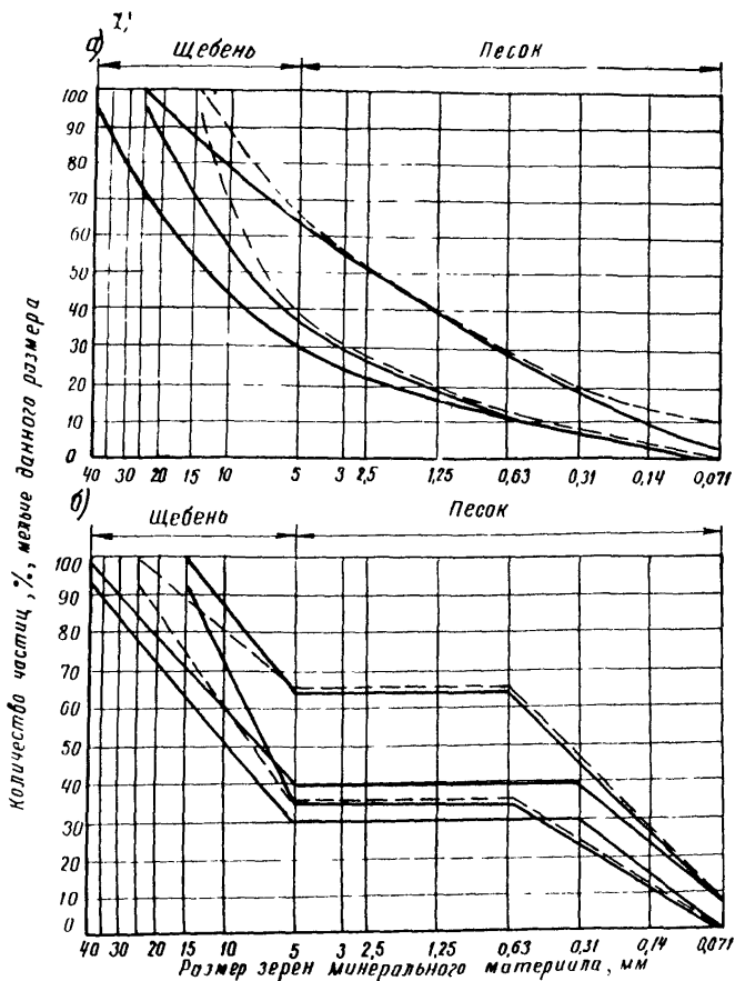
Рис.2. Зерновой состав минеральной части битумоминеральных смесей с непрерывной гранулометрией (а) и прерывистой (б)
