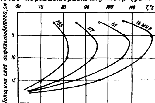
Рис.4. Температура асфальтобетонной смеси по толщине слоя в зависимости от времени после ее укладки (цифры на кривых — время после укладки)
