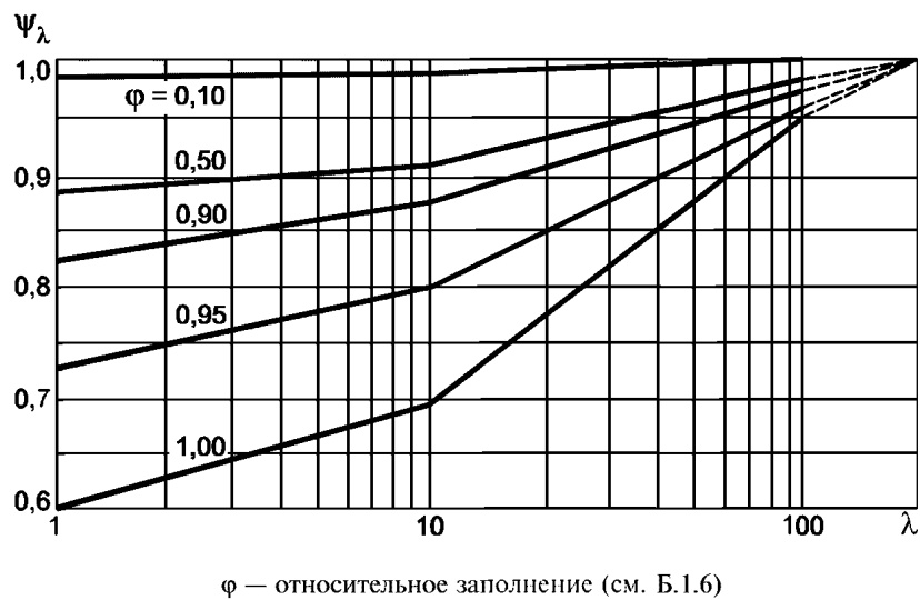
Рисунок Б.5 — Коэффициент \phi_\lambda , учитывающий относительное удлинение \lambda плоских и пространственных ферм ( \lambda = l / b ), (см. рисунок Б.4)
