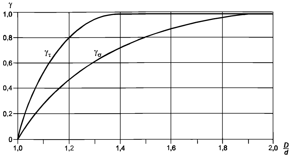
Рисунок И.1 — График для определения значений коэффициентов \gamma в формуле (И.1)
