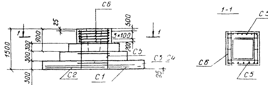
Армирование фундамента
