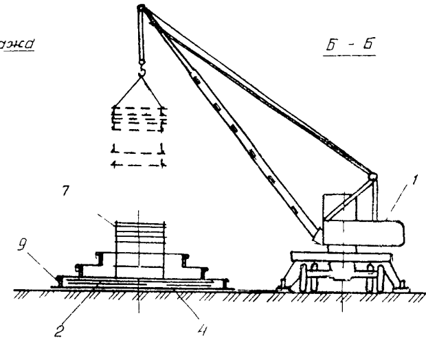
Схема установки фиксаторов
