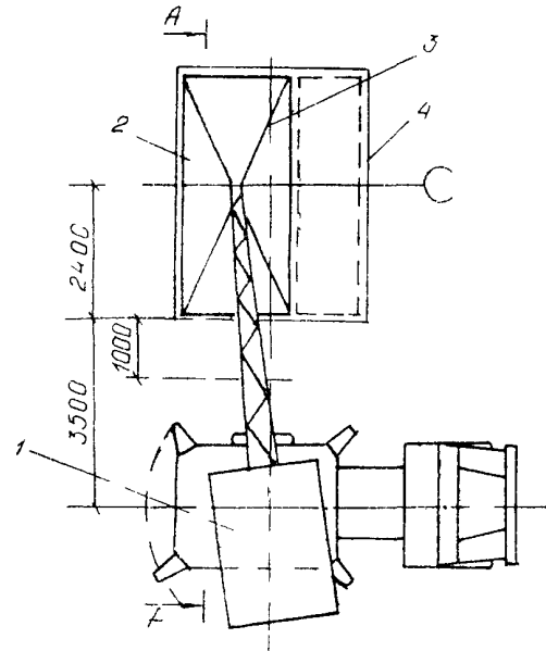
Схема монтажа арматурных сеток
