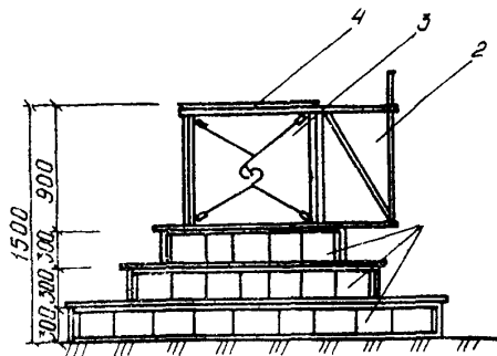
Стальные опалубочные формы для фундамента ВФ 14-01
