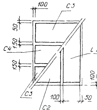
Схема раскладки сеток подшвы
