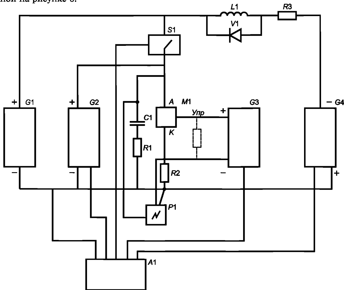
S1 — ключ; G1 — источник импульсов тока в открытом состоянии; G2 — источник импульсов повторяющегося напряжения; G3 — источник импульсов управления; G4 — источник импульсов обратного напряжения; R3 , L1 , V1 — резистор, катушка индуктивности и диод — соответственно цепи формирования импульсов источника G4 ; R2 — безындуктивный измерительный резистор; C1 , R1 — конденсатор и резистор — соответственно цепи защиты от перенапряжений; P1 — осциллограф; A1 — синхронизирующее устройство; M1 — тиристорный модуль
