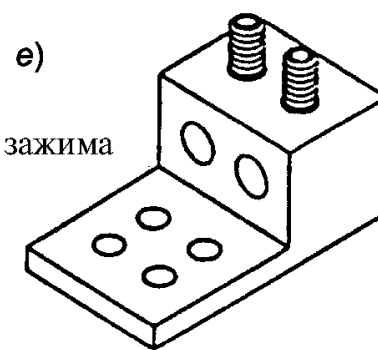
Рисунок F.3 — Торцевые зажимы с непосредственным зажимом проводника(ов)
