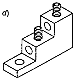
Рисунок F.3 — Торцевые зажимы с непосредственным зажимом проводника(ов)
