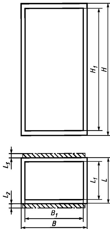
Рисунок 5 — Координационные размеры БНКЗ (корпус шкафа)
