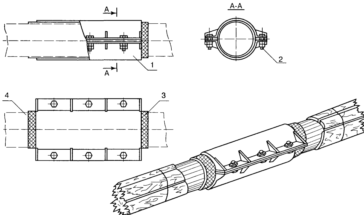
Рисунок 5 Зажим разъемный:
