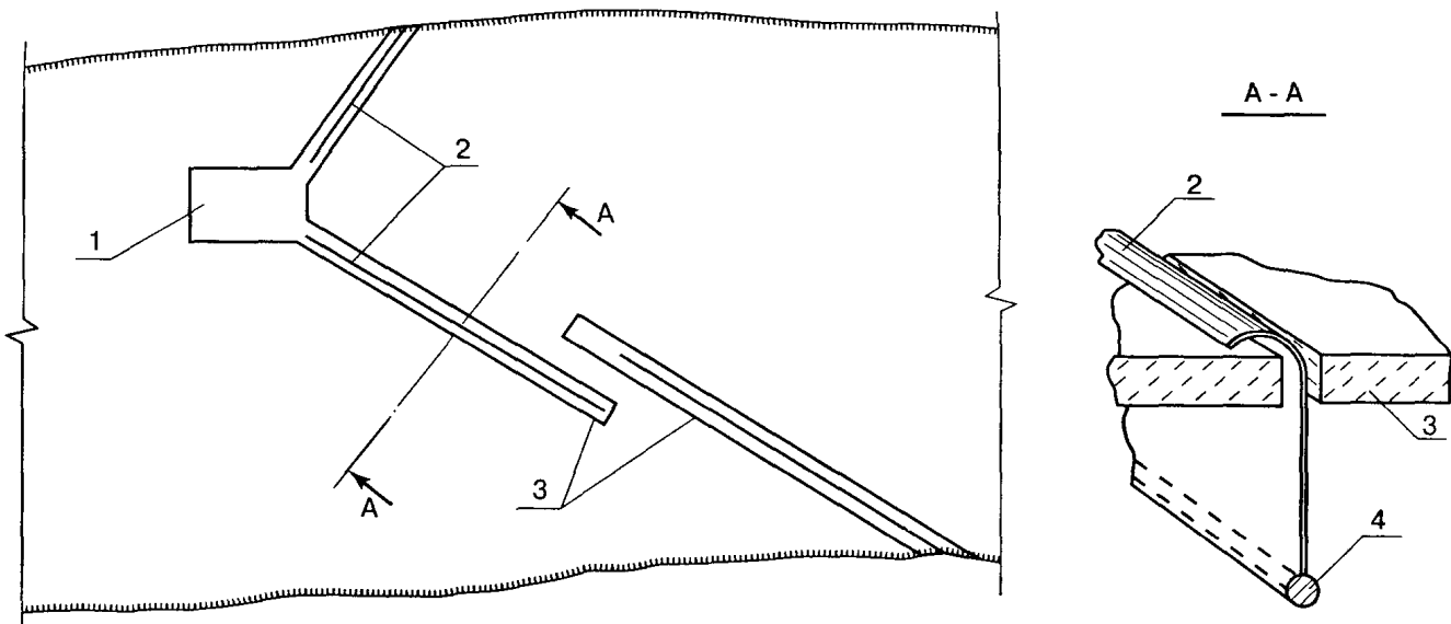
Рисунок 10. Схема локализации и направления пятна нефтепродукта в зимних условиях:
