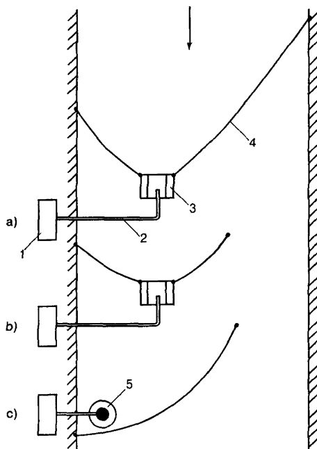
Рисунок 9. Схема установки ВЗ и НМСБ в потоке: 1 — емкость для сброса нефтепродуктов; 2 — отводящий рукав; 3, 5 — нефтесборщики; 4 — боновое заграждение
