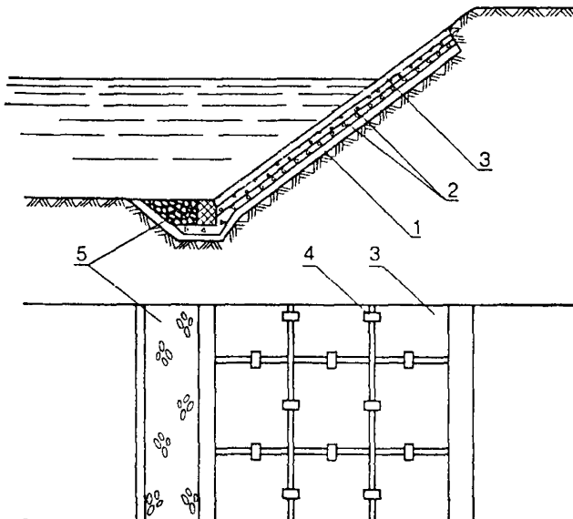
Рис. Б.9. Укрепление откосов плитами:
