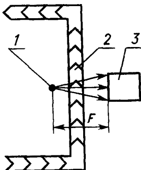
1—источник; 2—объект контроля; 3—дозиметр
