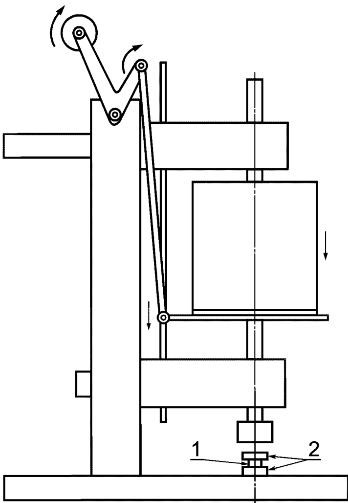
1 — образец; 2 — стеклянные пластины
