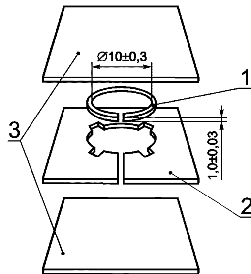
1 — разъемное кольцо, 2 — удерживающая пластина, 3 — покровные пластины
