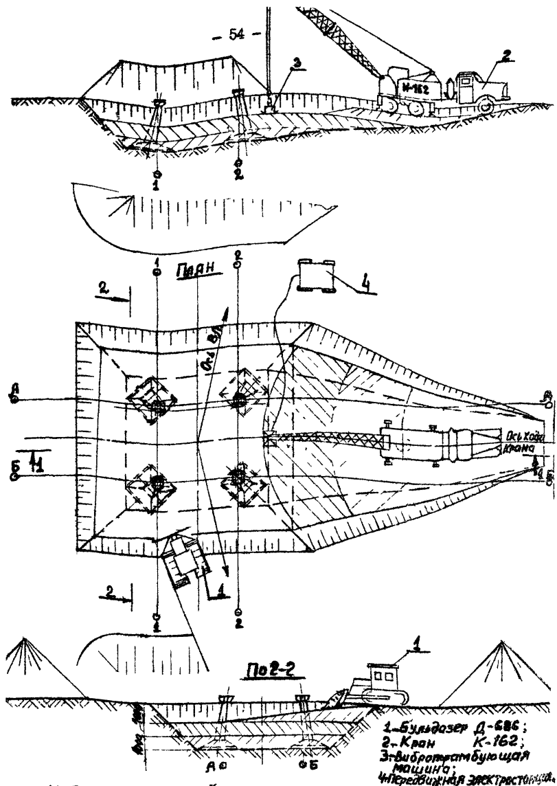
Рис. 11. Схема обратной засыпки котлованов под фундаменты аппаратов 4220-1; 4220-3; 4330-1; 4220-2; 4330-2.
