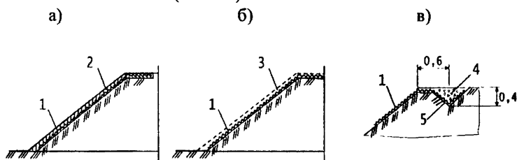
Рис. 7.1. Укрепление откосов земляного полотна биологическими типами укрепления с применением геосинтетических материалов:
