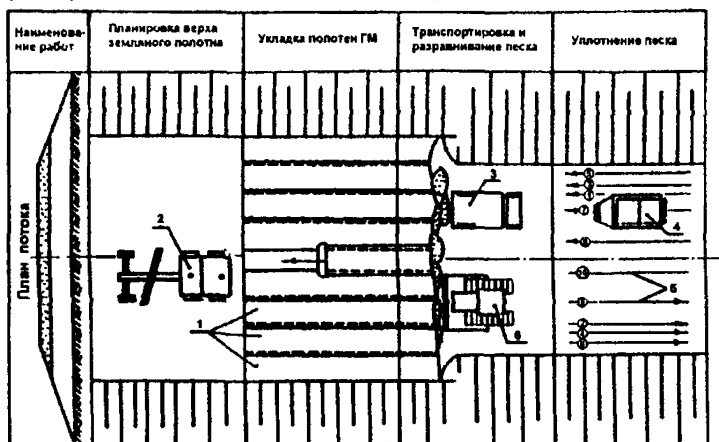
Рис. 5.9. Технологическая схема по устройству защитных (дополнительно – дренажных) прослоек из ГМ Геокот Д под песчаным подстилающим слоем дорожной одежды:
