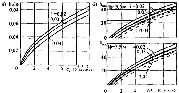
Рис 5.6. Номограмма к расчету дренирующего слоя по п. 5.2.4 (определение h_{\text{нас}} и C ): -пески средней крупности; - - - - - пески мелкие
