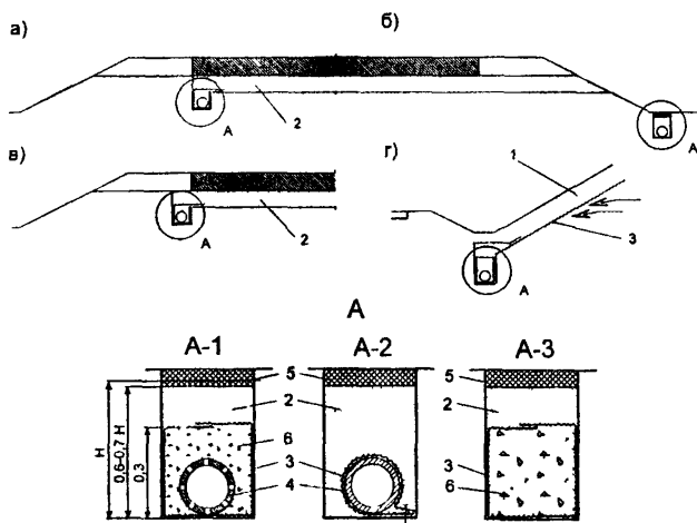
Рис. 6.1. Конструкции продольных дренажей с применением геотекстильных материалов:
