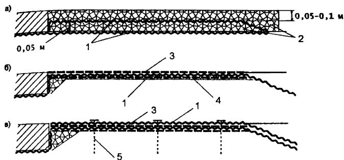
Рис . 6.4. Конструкция укрепления русел у водопропускных труб: 1 – геотекстильный материал; 2 – каменная наброска; 3 – розлив битума; 4 – обработанный щебень; 5 - анкер
