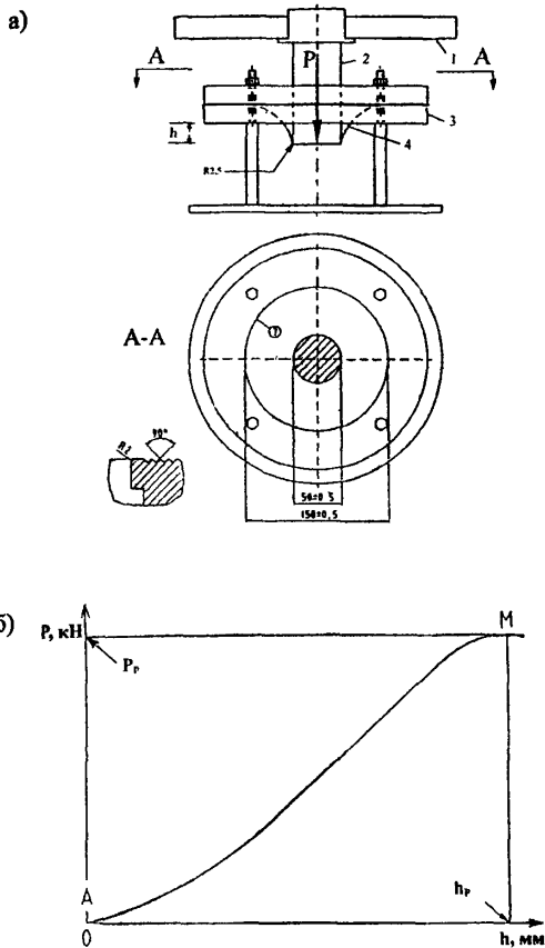
Рис. п.2.2. Определение механических характеристик ГМ на продавливание:
