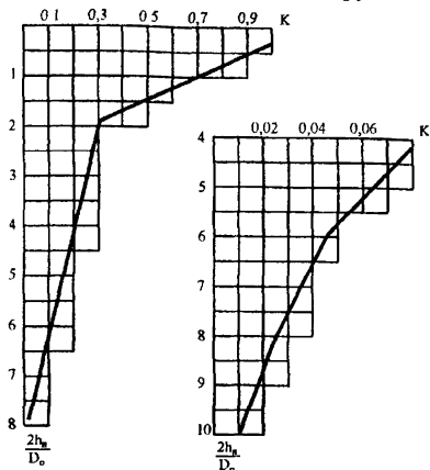
Рис. 4.8. Зависимость коэффициента распределения напряжений K от относительной глубины \frac{2h_n}{D_0}
