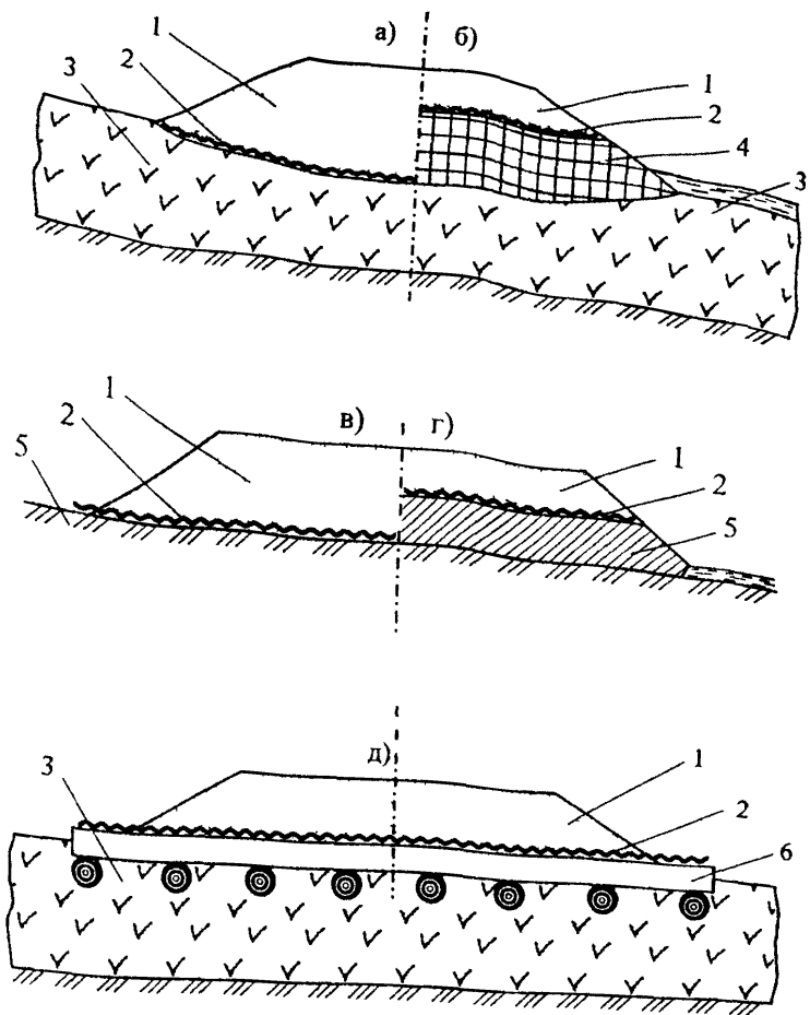
Рис. 4.2. Схемы конструкций временных дорог на слабых грунтах с геотекстильной прослойкой:
