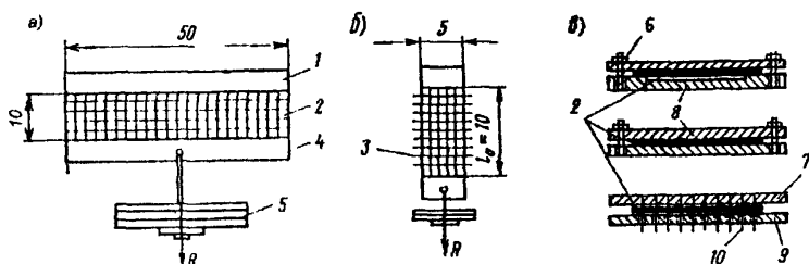
Рис. п 2.3 Схемы испытаний по методу длительного растяжения: 1,4 – зажимы, 2 – ГМ; 3 – накладки, 5 – грузы, 6 – стяжка; 7,8 – верхняя и нижняя накладки; 9 – накладка с отверстием под шпиль, 10 – шпиль
