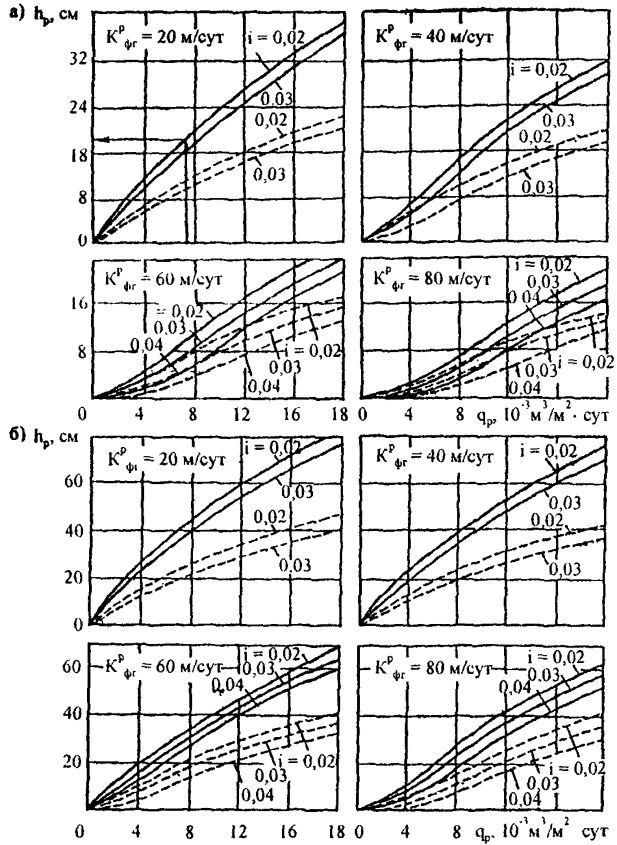
Рис. 5.5. Номограмма по расчету по п. 5.2.4 (определение h_p ): а – при l_{\phi} = 3,5\text{м} ; б – при l_{\phi} = 7,0\text{м} ; - при K_{\phi}^p = 1 ; при K_{\phi}^p = 3 \text{ м/сут}
