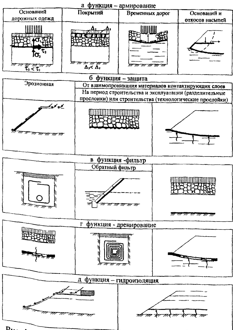
Рис 11 Основные функции геосинтетических материалов в дорожных конструкциях
