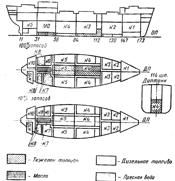
Расположение запасов на 6000 миль*
