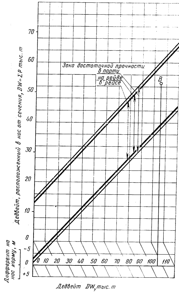
В сечении по 136 шп.
