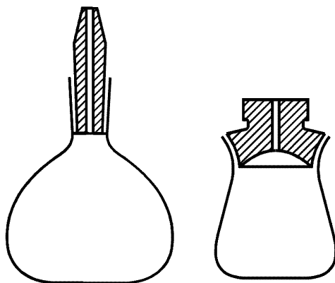
Рисунок 1 — Пикнометры
