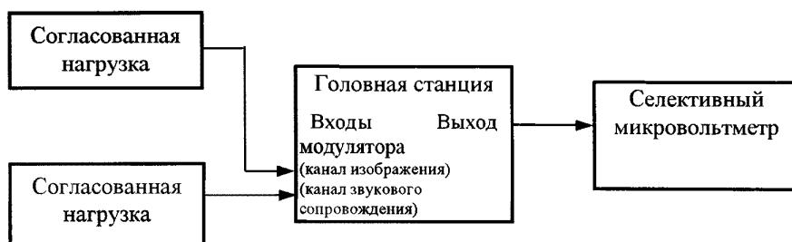
Рисунок 7.19 — Структурная схема для определения отношения радиосигнала изображения к побочным помехам, разности уровней напряжения радиосигналов изображения и звукового сопровождения, отношения радиосигнала изображения к шуму в полосе частот канала изображения
