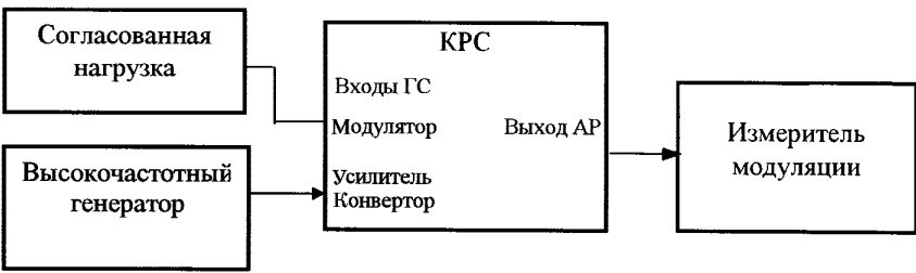
Рисунок 7.6 — Структурная схема для определения отношения сигнала изображения к фоновой помехе
