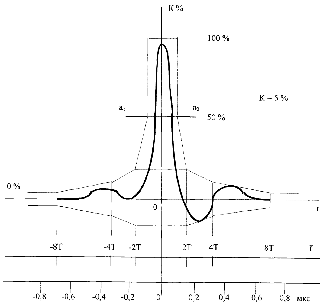
Рисунок 7.3 — Осциллограмма 2Т-импульса измерительного сигнала № 2 (ГОСТ 18471)
