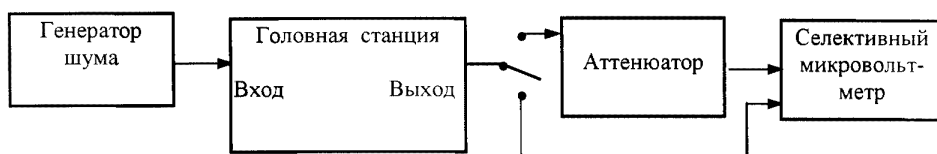
Рисунок 7.10 — Структурная схема для измерения коэффициента шума
