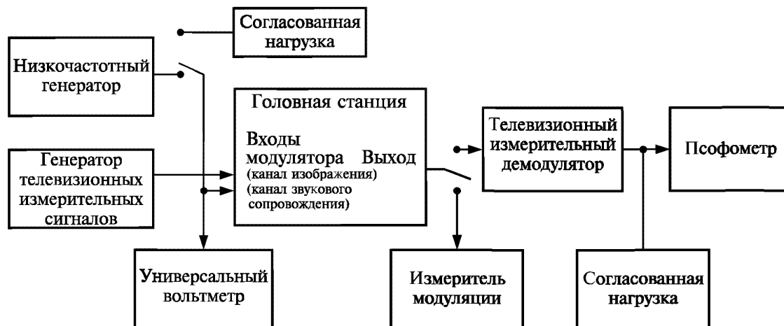
Рисунок 7.28 — Структурная схема для определения отношения сигнала звукового сопровождения к шуму
