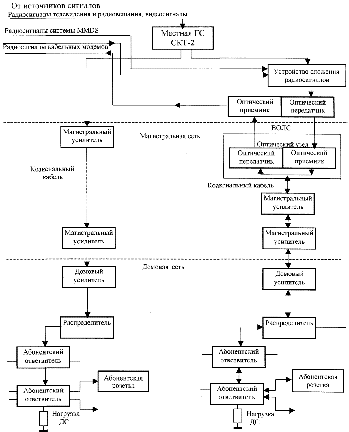
Рисунок 4.2 — Структурные схемы районной кабельной распределительной сети СКТ-2
