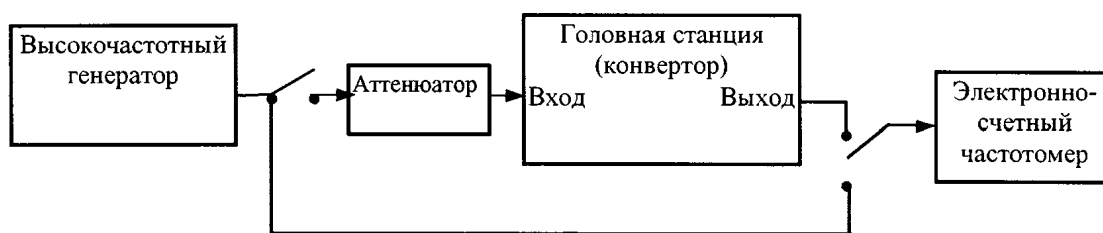
Рисунок 7.16 — Структурная схема для определения отклонения от номинального значения несущей частоты радиосигналов изображения и ОВЧ ЧМ вещания
