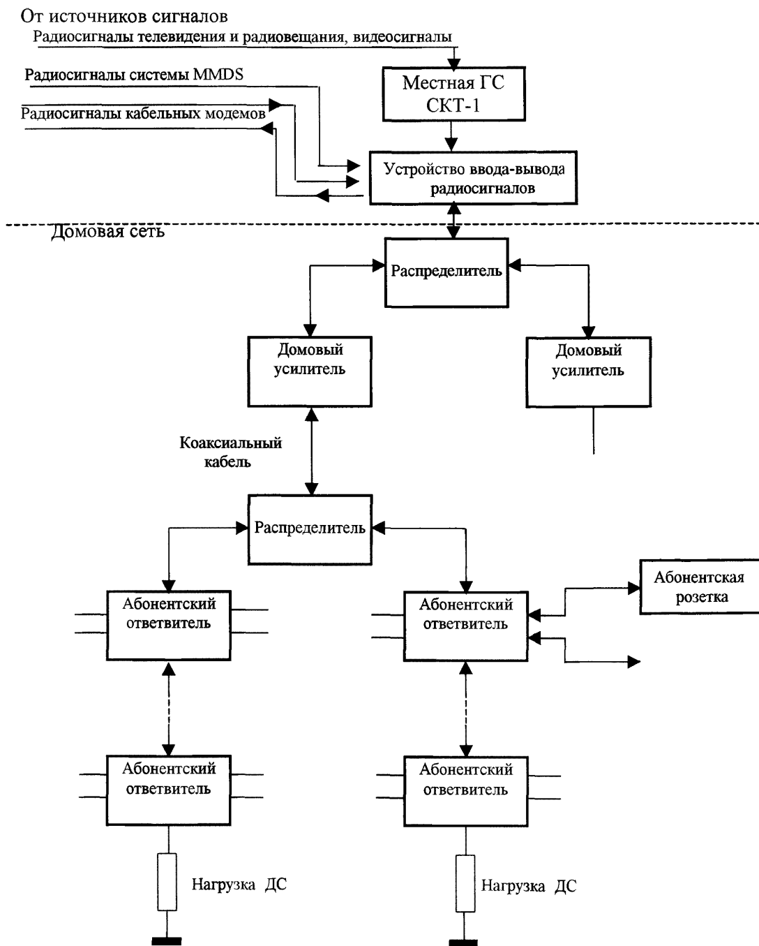
Рисунок 4.1 — Структурная схема местной кабельной распределительной сети СКТ-1
