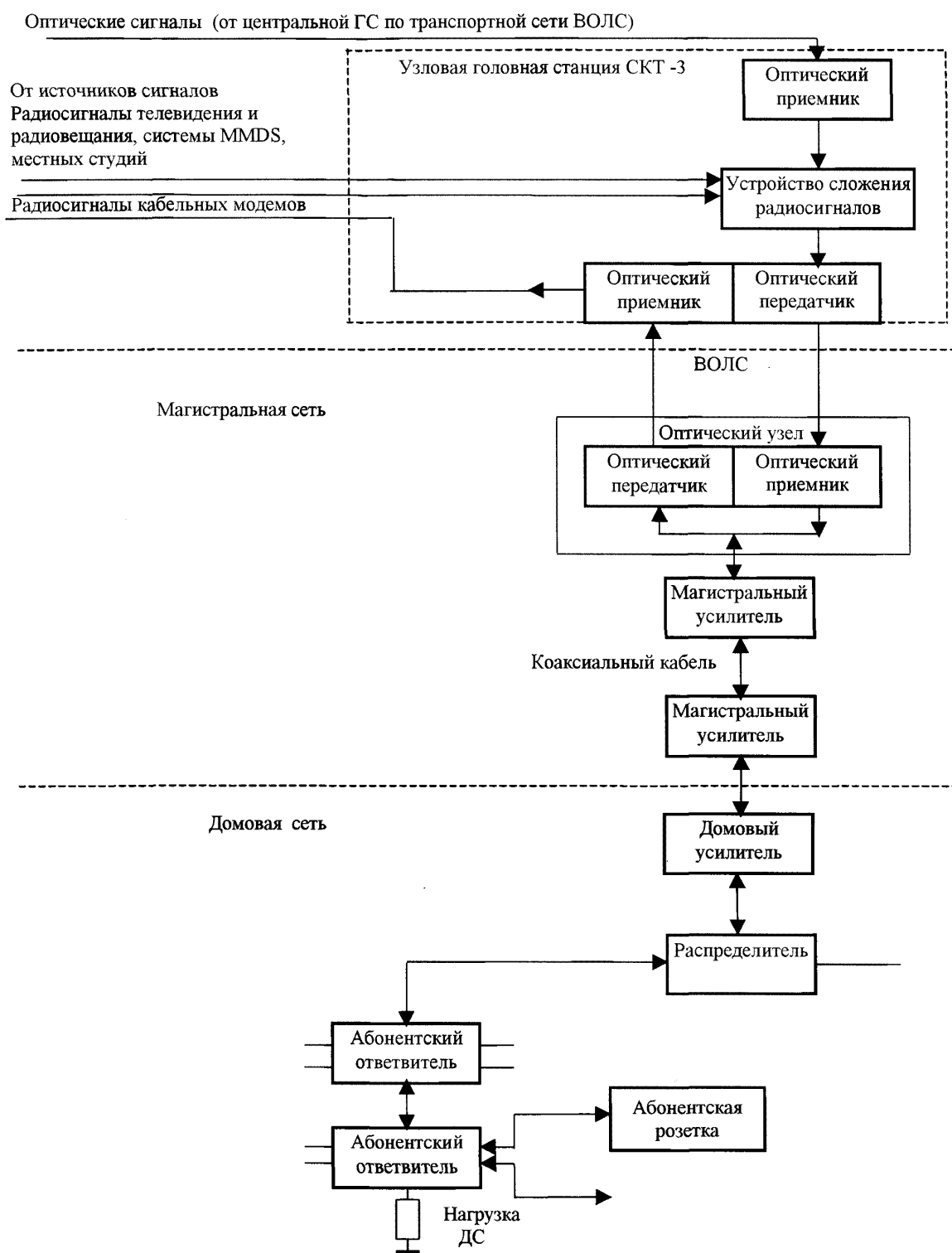
Рисунок 4.3 — Структурная схема городской кабельной распределительной сети СКТ-3
