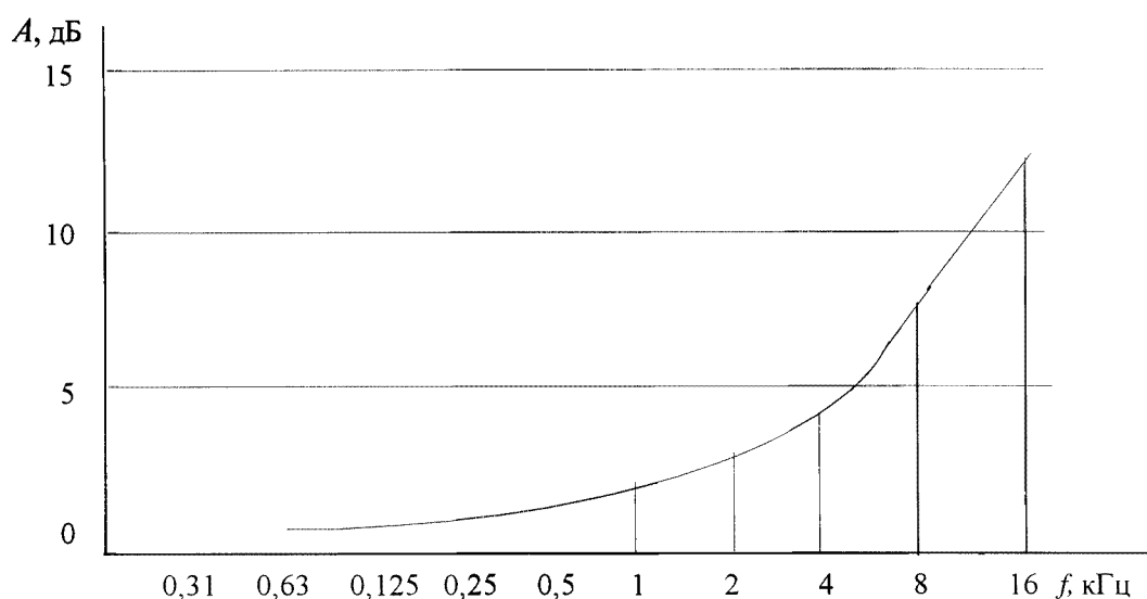
Рисунок 5.2 — АЧХ цепи предискажения с постоянной времени 50 мс
