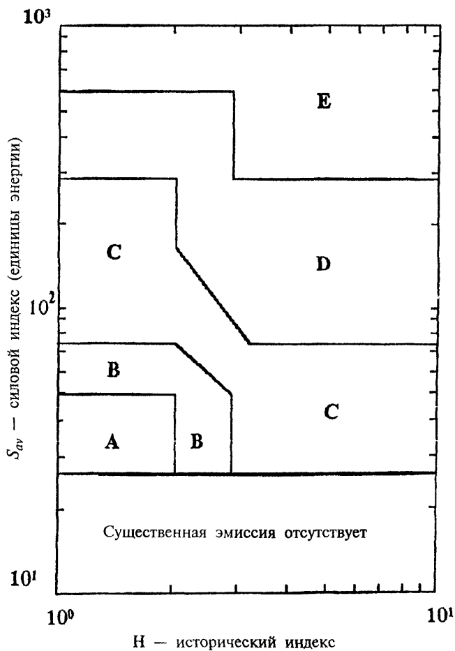
Диаграмма классификации источников АЭ в технологии MONPAC
