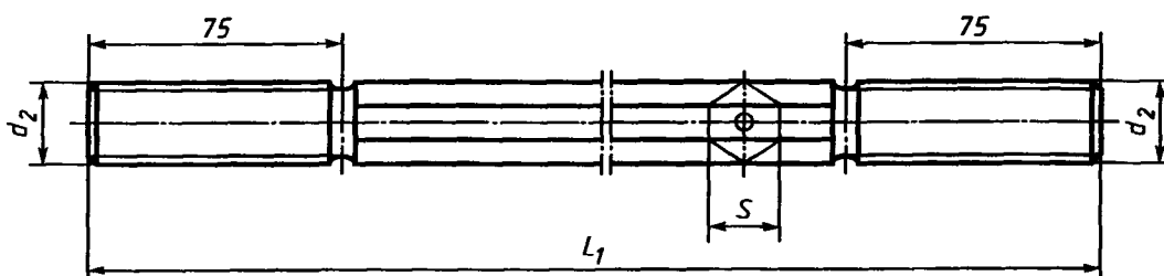
Рисунок 5 — Буровые и удлинительные штанги с резьбой
