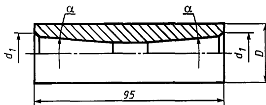
Рисунок 3 — Соединительная муфта
