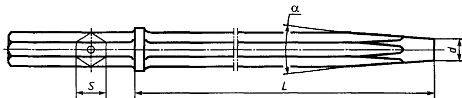
Рисунок 1 — Буровые штанги с конусом
