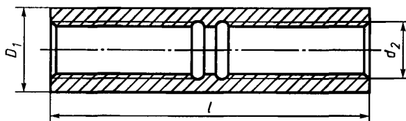
Рисунок 6 — Соединительная муфта
