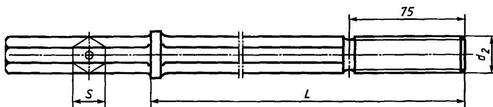
Рисунок 4 — Буровые штанги с резьбой
