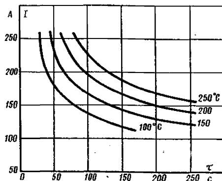
Рис.13. Зависимость нагрева провода ПС-25 от режима плавки
