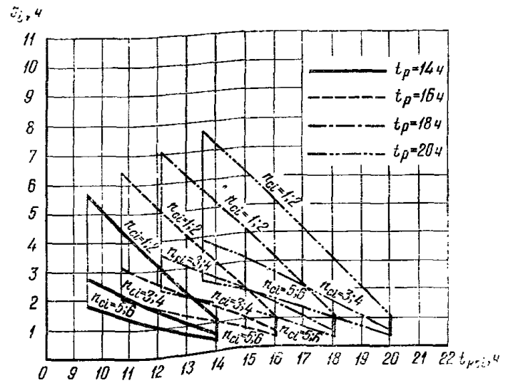
Рис. 2. График для определения основного значения I_i при \frac{2}{3} t_p < t_{крп} \leq t_p
