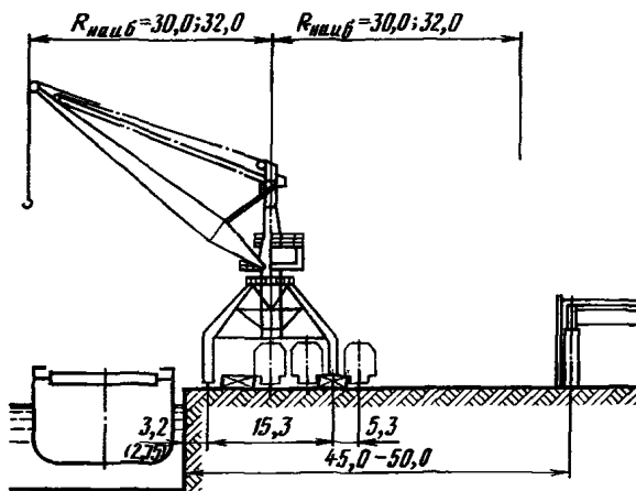
Вариант с тремя прикордонными железнодорожными путями
