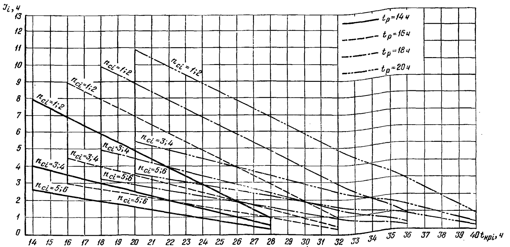
Рис. 3. График для определения основного значения I_i при t_p < t_{крп} \leq 2t_p
