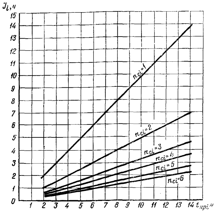
Рис. 1. График для определения основного значения I_i при t_{крп} < \frac{2}{3} t_p
