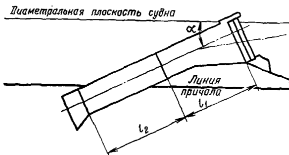
Рис. 5. Возвышение кордона для судна с угловой рампой без груза при расчетном высоком уровне воды
