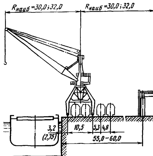
Вариант с четырьмя прикордонными железнодорожными путями
