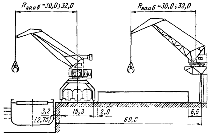
Вариант с тремя прикордонными железнодорожными путями
