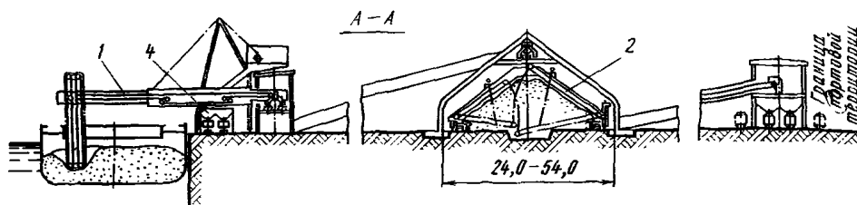
Вариант склада для слеживающихся грузов
