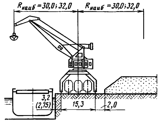
Вариант с тремя прикордонными железнодорожными путями
