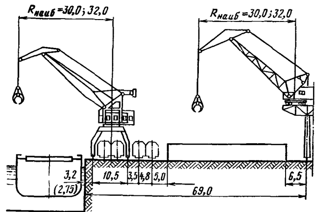
Вариант с четырьмя прикордонными железнодорожными путями
