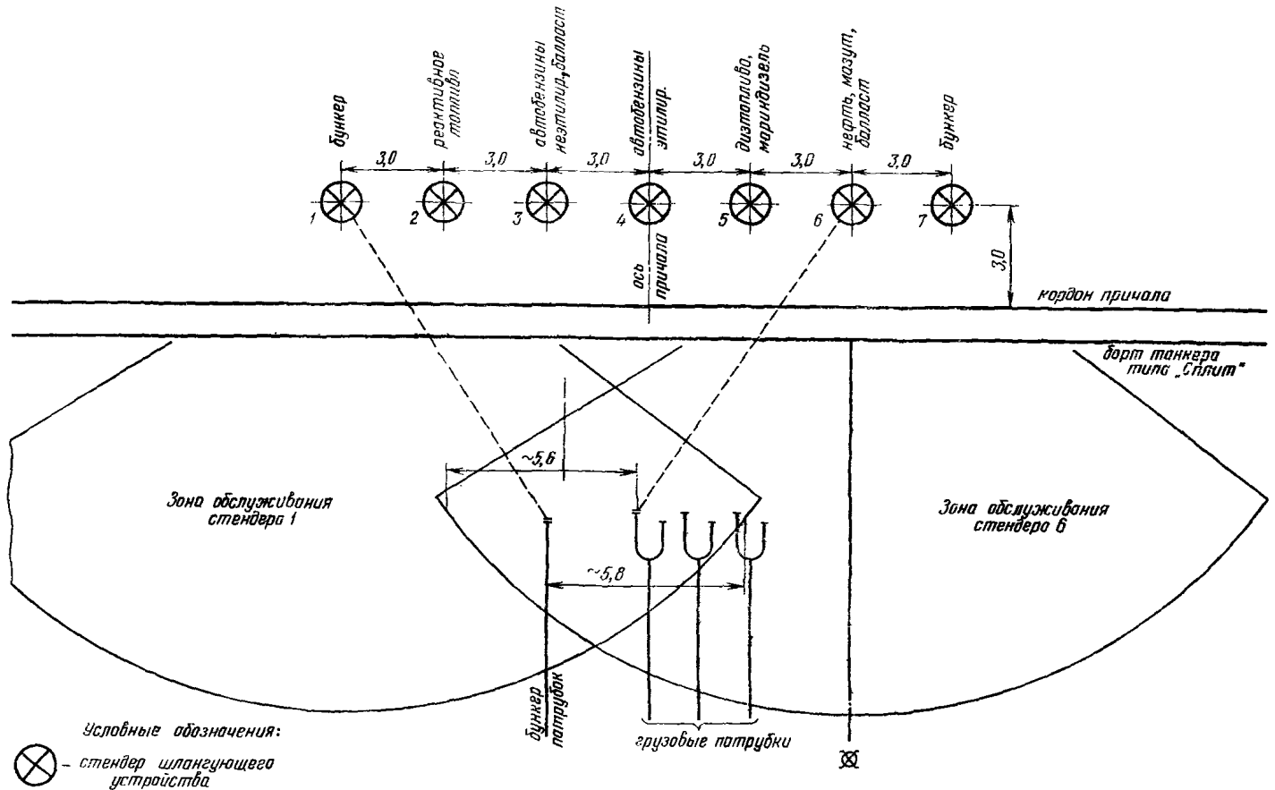
Рис. 1. Схема совмещения зон обслуживания стендеров с зоной расположения судовых приемно-отливных патрубков
