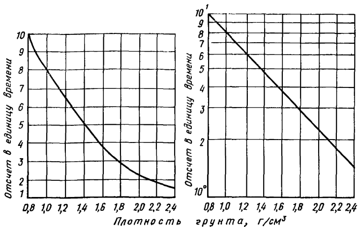
График градуировки радиоизотопного плотномера (тип. №)
