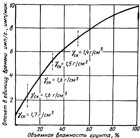
График градуировки нейтронного влагомера
