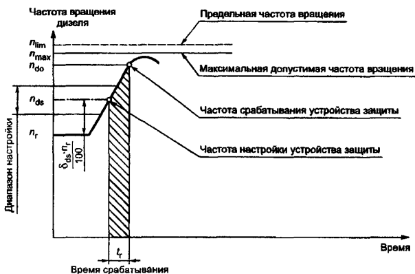
Рисунок 1 — Типичная кривая срабатывания устройства защиты
