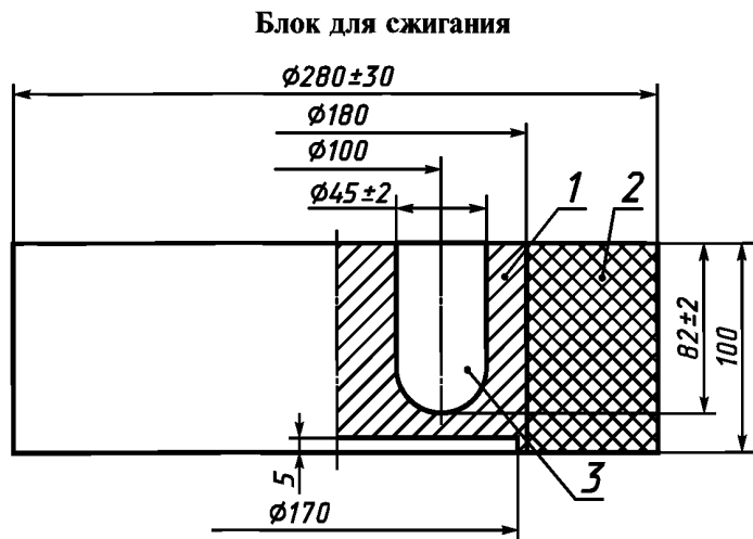
Рисунок А.1 — Алюминиевый блок с шестью гнездами
