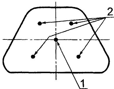
1 — центр тяжести полного сечения; 2 — центры тяжести каждой части сечения
