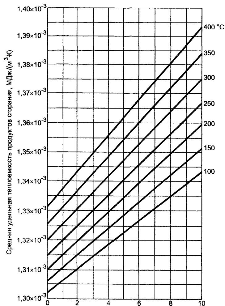
Рисунок 11 — Средняя удельная теплоемкость продуктов сгорания
