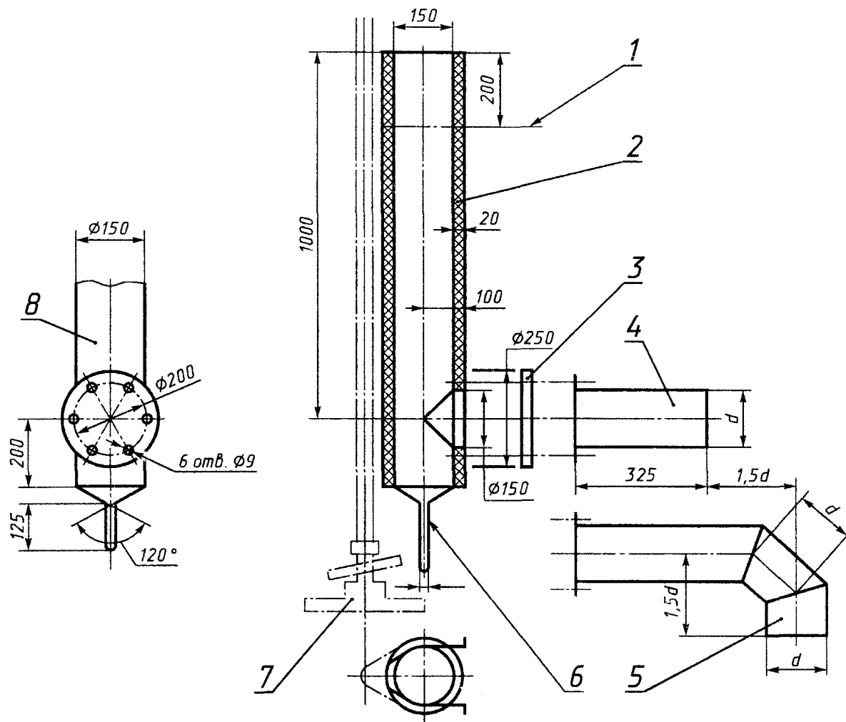
1 — плоскость измерения (пробоотборник и термопара); 2 — теплоизоляция (стекловолокно плотностью 64 \text{ кг/м}^3 ); 3 — прокладка; 4, 5 — соединительные трубы из нержавеющей стали; 6 — трубка внутренним диаметром 8 мм и толщиной стенки 1 мм; 7 — опорная стойка (высота регулируемая); 8 — труба дымохода из нержавеющей стали
