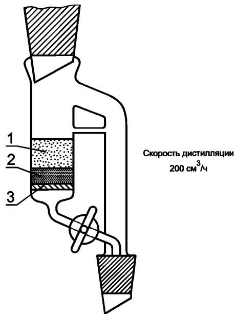
1 — табак + Флоризил®; 2 — флоризил®; 3 — пористая фильтрующая пластина № 1 размером пор 100—120 мкм
