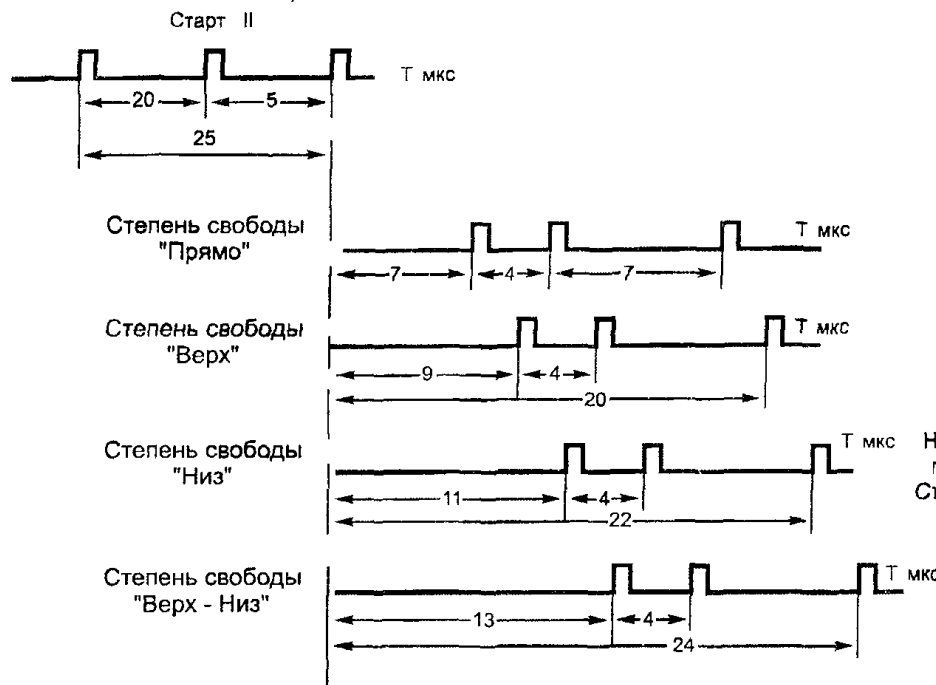
б) Расположение сигнала "Стоп СС"
