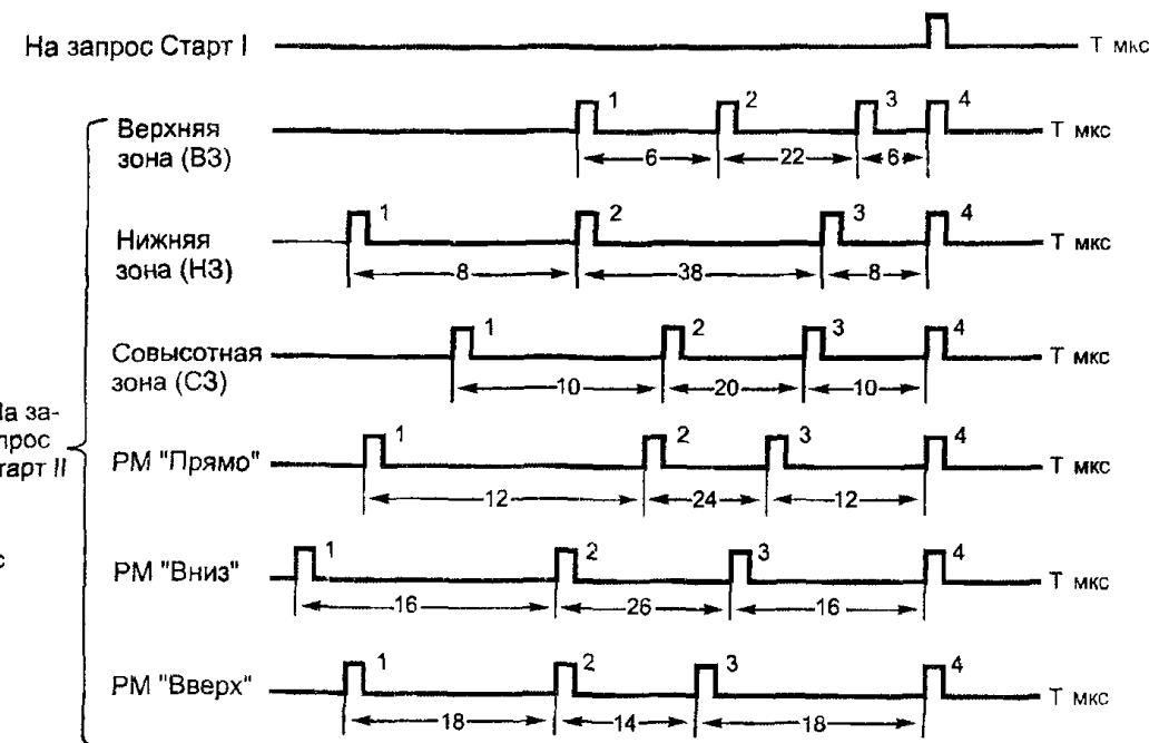
в) Структура ответных сигналов
