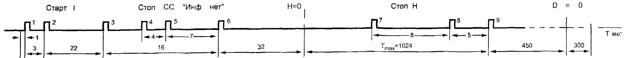
б) Расположение сигнала "Стоп СС"
