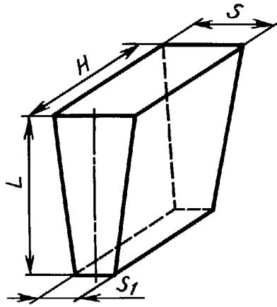
Рисунок 5 — Клин торцовый полуторный двусторонний
