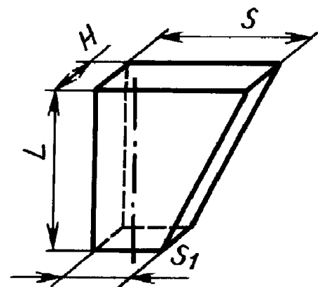
Рисунок 8 — Клин трапецеидальный односторонний
