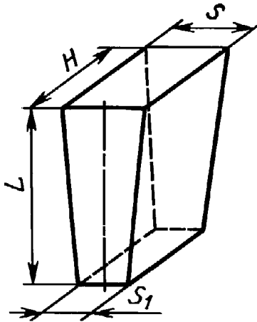
Рисунок 3 — Клин торцовый двусторонний
