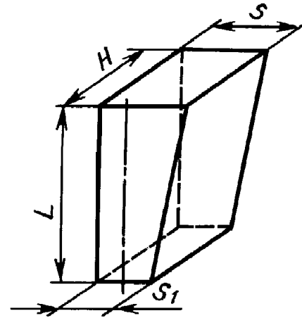
Рисунок 4 — Клин торцовый односторонний
