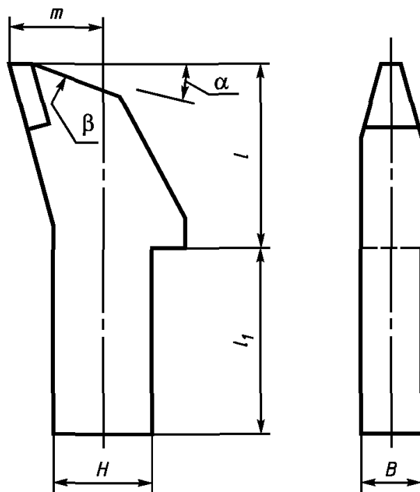
Рисунок 1 — Резец типа Р
