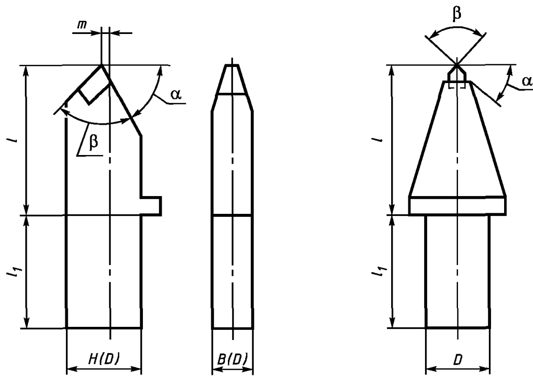
Рисунок 2 — Резец исполнения ТН
