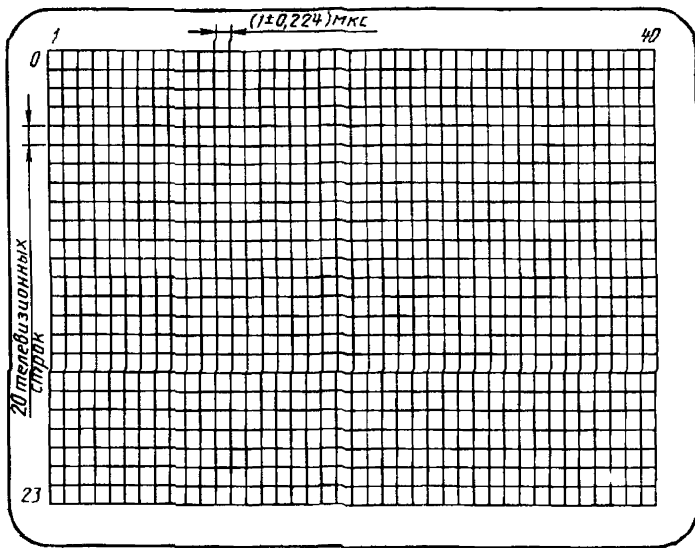
Рисунок 4 — Расположение знакомест на странице телетекста
