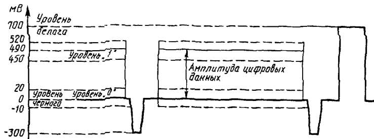
Рисунок 2 — Уровни сигнала цифровых данных сигнала телетекста
