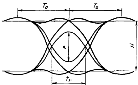
Рисунок 10 — Осциллограмма глазковой диаграммы
