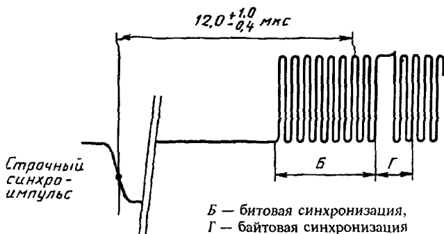
Рисунок 3 — Синхронизация сигнала цифровых данных телетекста
