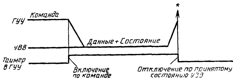
Временная диаграмма для команд чтения
