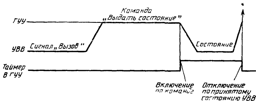
Временная диаграмма обработки сигнала «Вызов»
