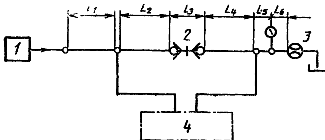
Принципиальная схема испытательной установки
