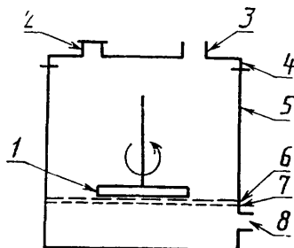
Условное изображение ячейки для определения производительности мембран
