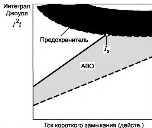
Ток короткого замыкания (действ.)
