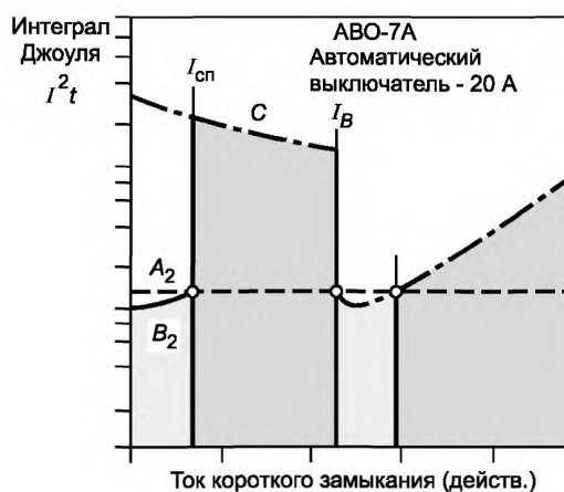
Рисунок F.8 — Примеры подлинной и ошибочной координации
