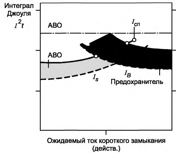
Рисунок F.2 — АВО с тепловым расцепителем, резервной защитой, осуществляемой плавким предохранителем
