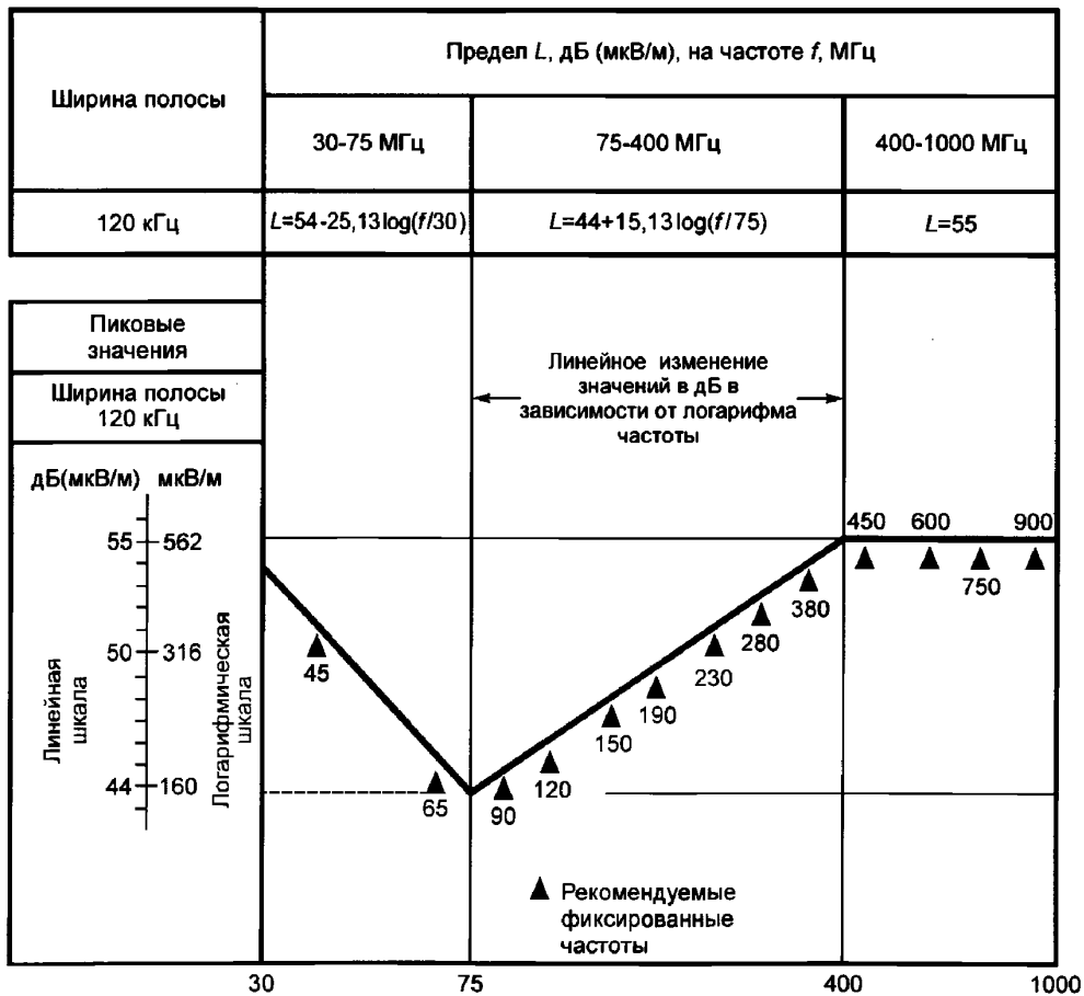
Частоты в мегагерцах — логарифмическая шкала (см. 6.6.2.1)
