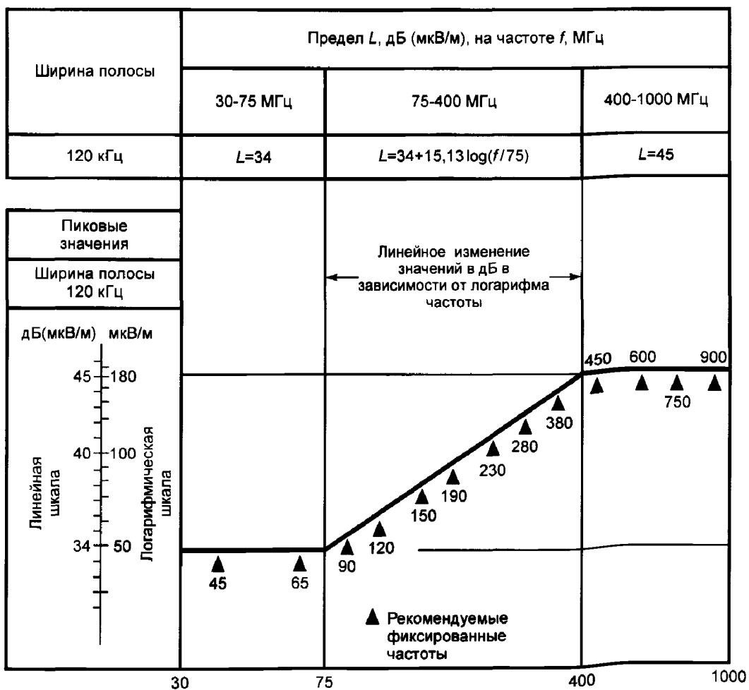
Частоты в мегагерцах — логарифмическая шкала (см. 6.3.2.2)
