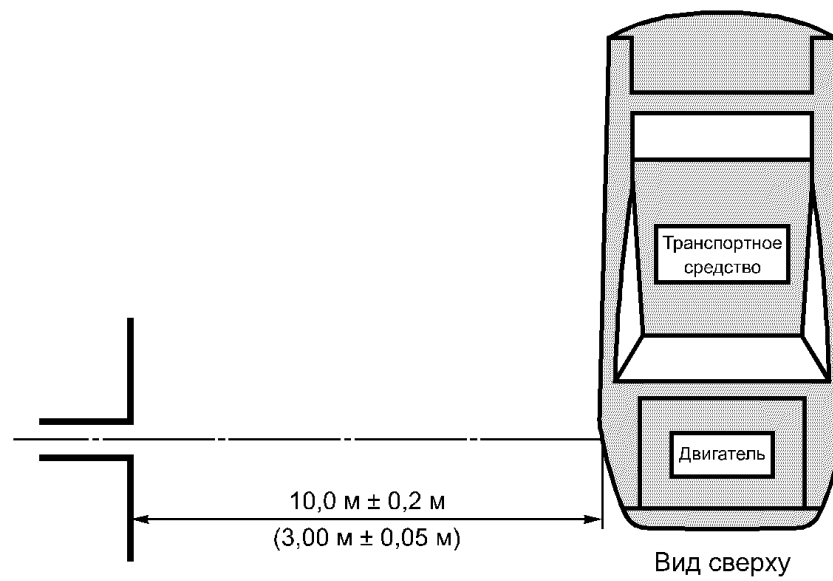
Рисунок 2 — Расположение антенн по отношению к транспортному средству
