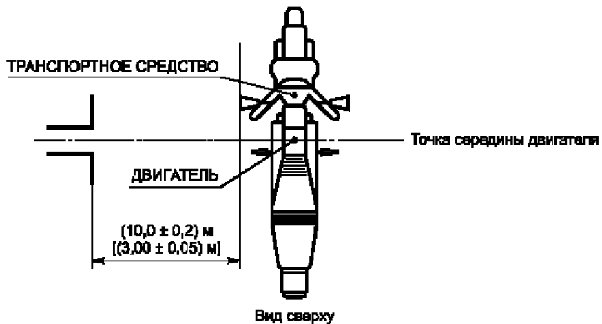
Рисунок 4 — Положение антенны по отношению к транспортному средству
