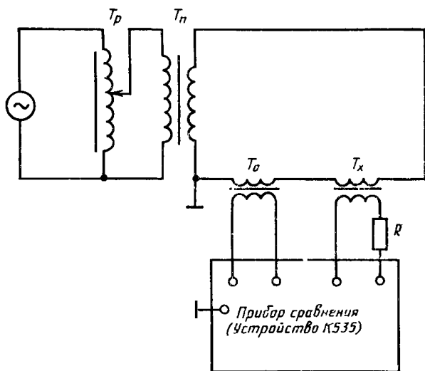
Схема для проверки трансформатора тока дифференциально-нулевым методом с использованием образцового трансформатора тока
