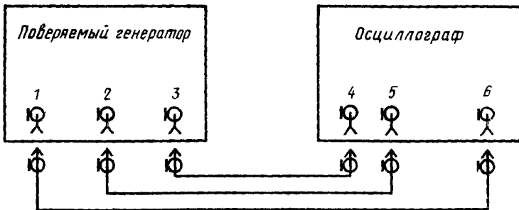
1—вход внешнего запуска; 2—выход синхронизирующих импульсов; 3—выход основных импульсов; 4—вход I канала Y; 5—вход II канала Y; 6—выход импульсов синхронизации
