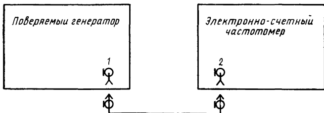
1—выход основных импульсов; 2—вход сигнала для измерения частоты и периода
