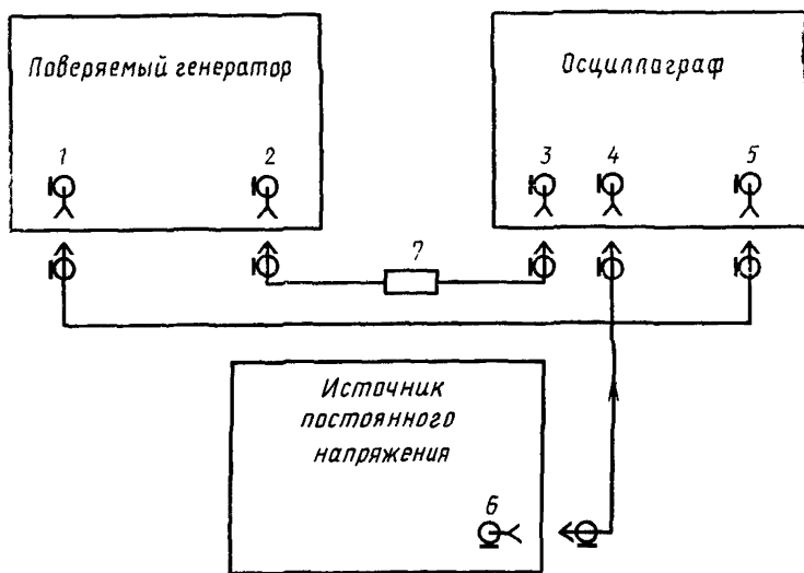
1—выход синхронизирующих импульсов; 2—выход основных импульсов; 3—вход 1 канала Y ; 4—вход II канала Y ; 5—вход синхронизирующих импульсов; 6—выход постоянного напряжения; 7—аттенюатор
