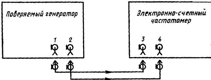
1—выход основных импульсов канала I; 2—выход основных импульсов канала II; 3—вход опережающего сигнала; 4—вход задержанного сигнала
