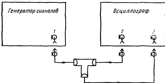
1—выход сигнала, 2—вход канала Y; 3—вход синхронизирующего сигнала Черт. 10
