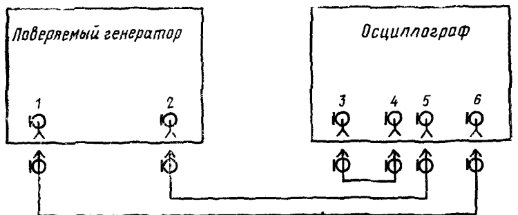
1—выход синхронизирующих импульсов, 2—выход основных импульсов, 3—выход сигнала калибратора напряжения, 4—вход I канала У, 5—вход II канала У, 6—вход синхронизирующих импульсов
