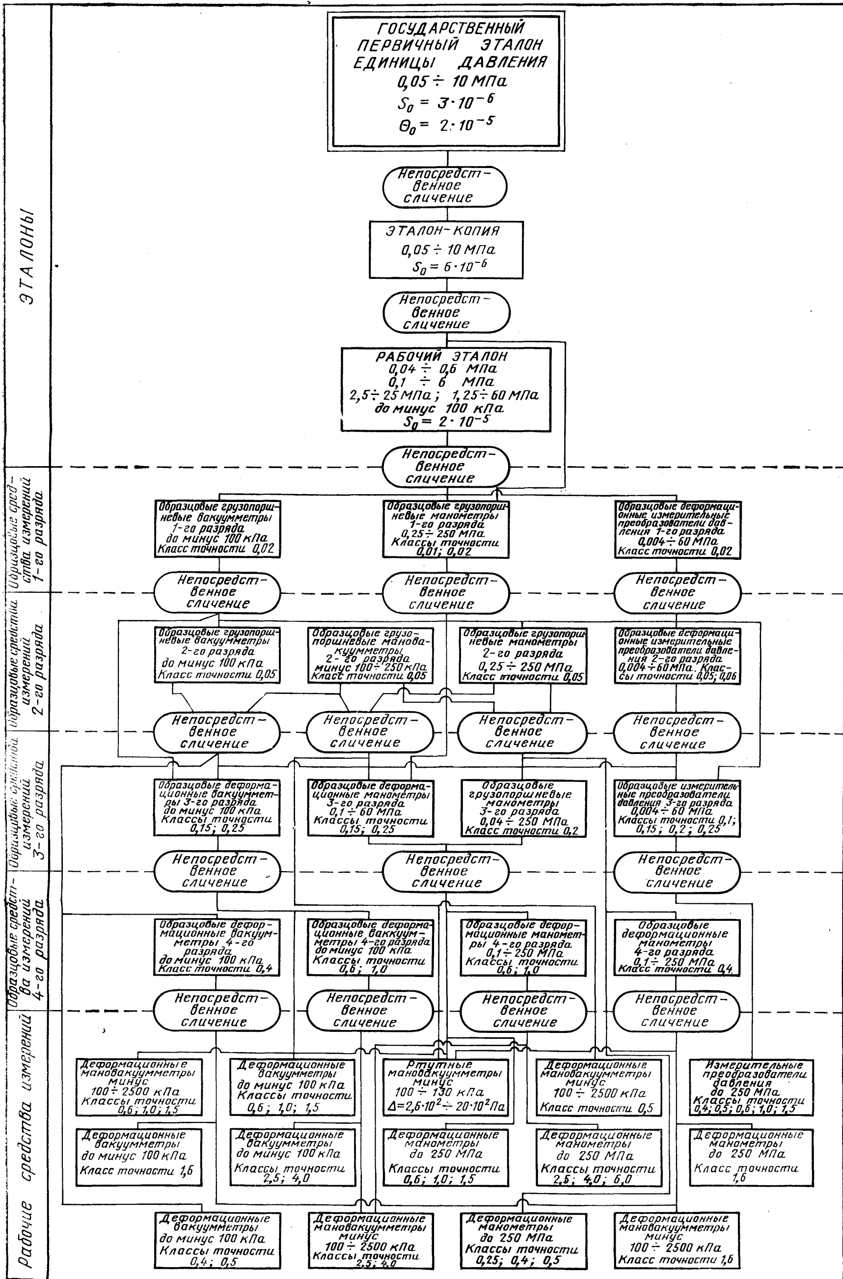
Общесоюзная поверочная схема для средств измерений избыточного давления до 250 МПа
