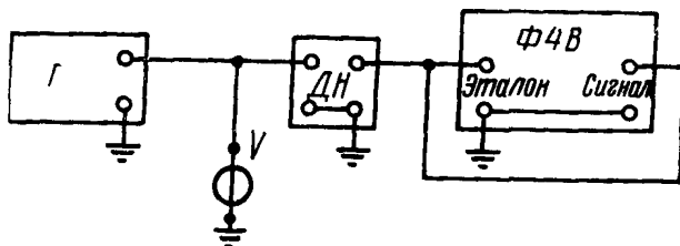
Г—измерительный генератор; V—образцовый вольтметр; ДН—безреактивный делитель напряжения, Ф4В—поверяемый фазочувствительный вольтметр.
