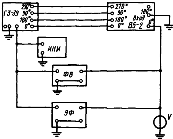
Схема проверки вольтметра В5—2
