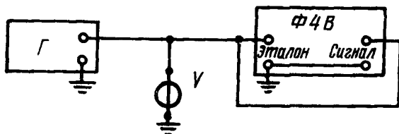
Г—измерительный генератор; V—образцовый вольтметр; Ф4В—поверяемый фазочувствительный вольтметр.
