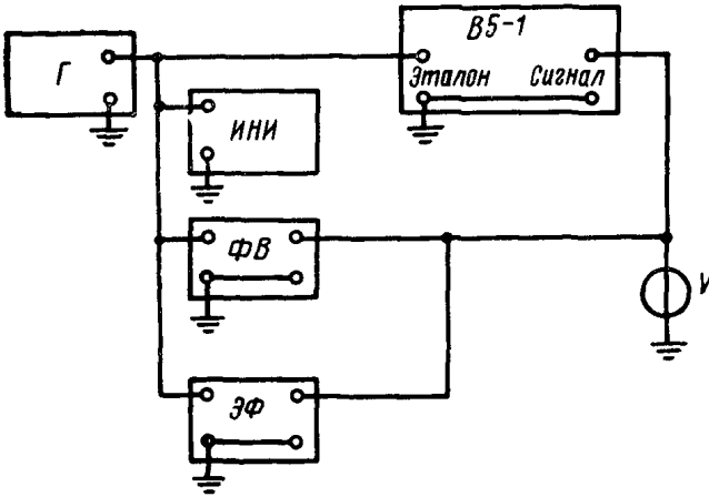
Схема проверки вольтметра В5—1
