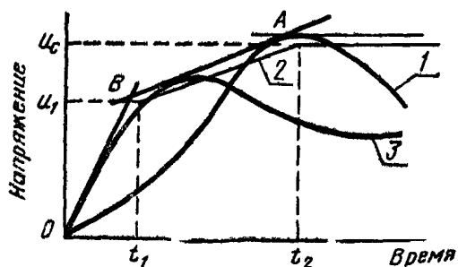
Кривые ПВН и их огибающие при двухэтапном испытании
