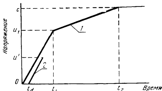
Характеристики ПВН
