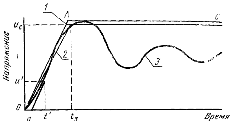
1—огибающая ПВН; 2—условная границная линия ПВН; 3—собственное ПВН
