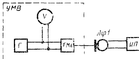
Г—звуковой генератор или генератор шума, V—вольтметр, ГМК—генератор механических колебаний; ИП—измерительный прибор (милливольтметр, измерительный усилитель, прибор для автоматической записи частотных характеристик, измеритель нелинейных искажений или схема, указанная на черт. 4, при измерении угольных ларингофонов; Лр1—ларингофон Черт. 6
