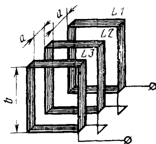
L1, L3 —катушки в 200 витков, L2 —катушка в 72 витка, a=75 мм — расстояние между катушками, b=200 мм—сторона квадрата каркаса.
