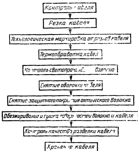
Схема технологического процесса разделки оптического кабеля
