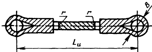
Машина для испытаний с кнехтами для наращенных петель (отметка r расположена на расстоянии 150 мм от последнего витка сращивания)
