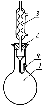
1 — колба; 2 — резиновая пробка; 3 — холодильник; 4 — градуированный приемник
