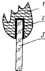
1—резиновый уплотнитель; 2—мастика, 3—стекло
