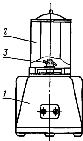
1—привод; 2—мерный стакан; 3—импеллер
