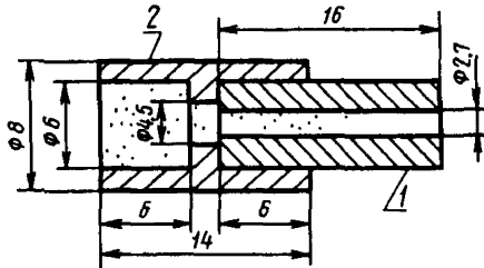
1 — нижняя часть электрода, зажимаемая в электродержателе; 2 — насадка
