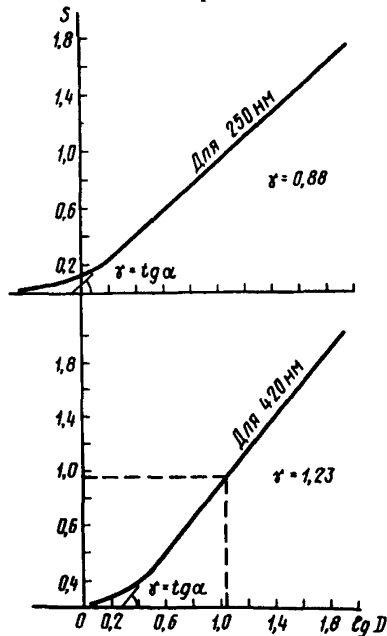
Характеристические кривые фотопластинок типа «Микро»
