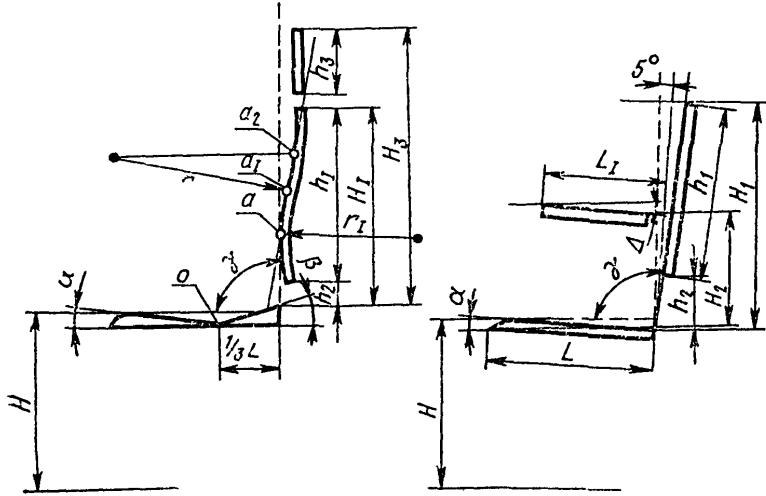
Кресло с непрофилированными элементами
