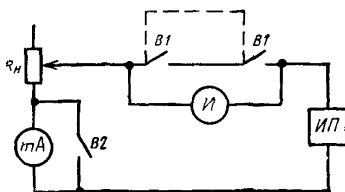
B1 —испытуемый выключатель; B2 —выключатель для защиты амперметра; И —индикатор; ИП —источник питания постоянного или переменного тока; мА —миллиамперметр; R_n —нагрузочный реостат
