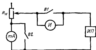
B1 —испытуемый выключатель; B2 —выключатель для защиты амперметра; И —индикатор; ИП —источник питания постоянного или переменного тока; мА —миллиамперметр; R_n —нагрузочный реостат
